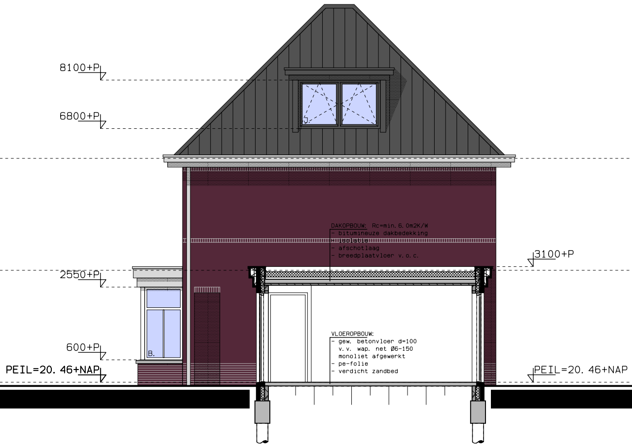
doorsnede C - C
